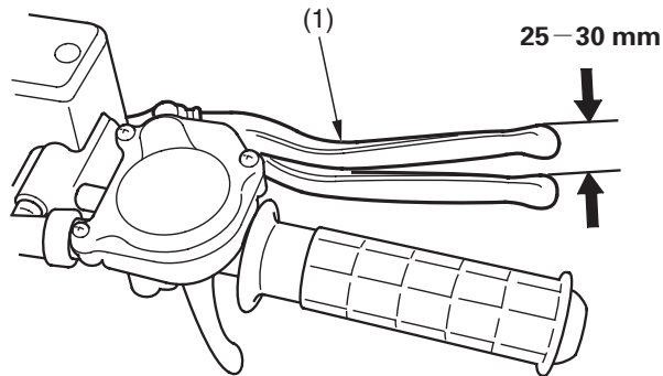
(1) etujarruvipu
