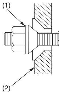
(2) vanne
